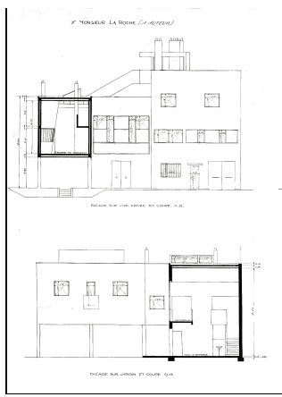
Maison La Roche
